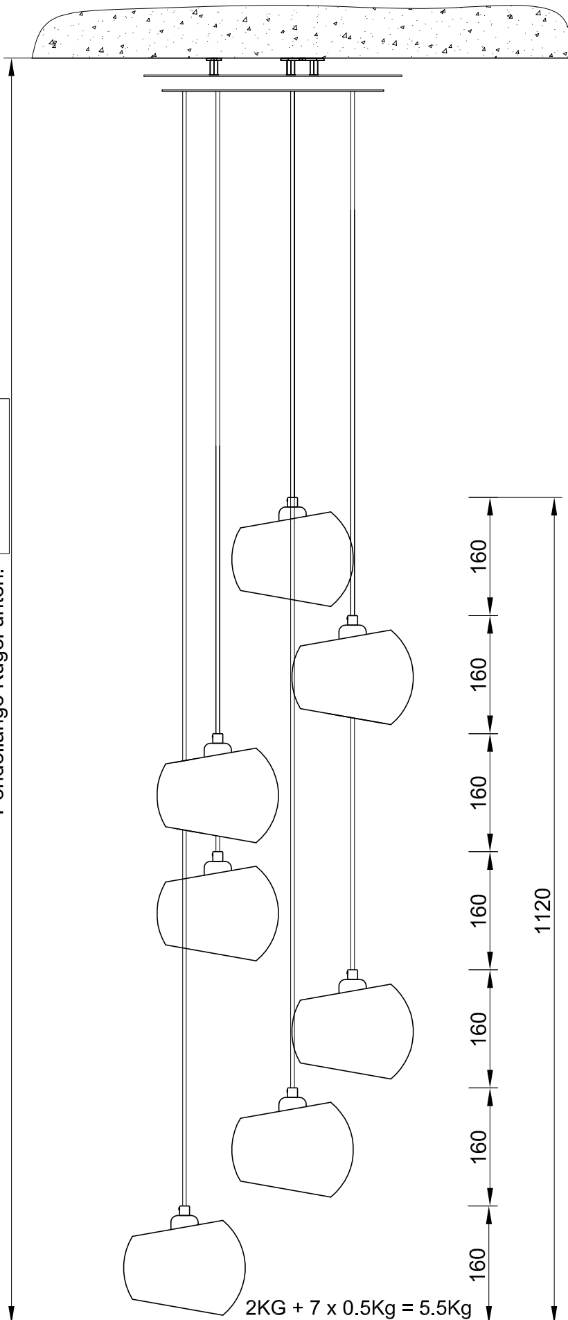
Kabellängen von der Fassung bis Baldachin (ohne Verdrahtung)
